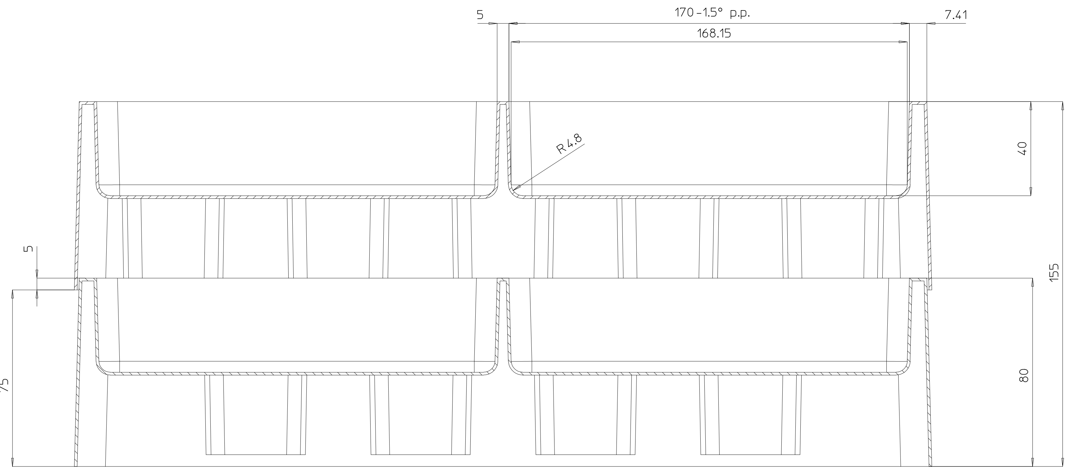
Sezione A-A
